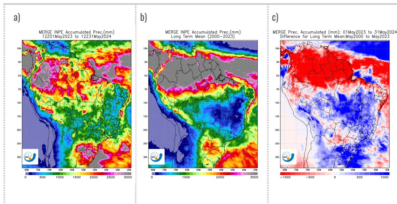
Figura 1.1.1: a) Acumulado de precipitação obtido pelo MERGE (um produto que combina dados de estações de superfície e estimativas por satélites) entre 1 de maio de 2023 e 31 de maio de 2024; b) Média de Longo Termo (MLT) acumulado de precipitação em maio entre 2000 e 2023; c) Diferença no acumulado de precipitação entre 1 de maio de 2023 e 31 de maio de 2024 vs. média de longo termo da precipitação (MLT).
