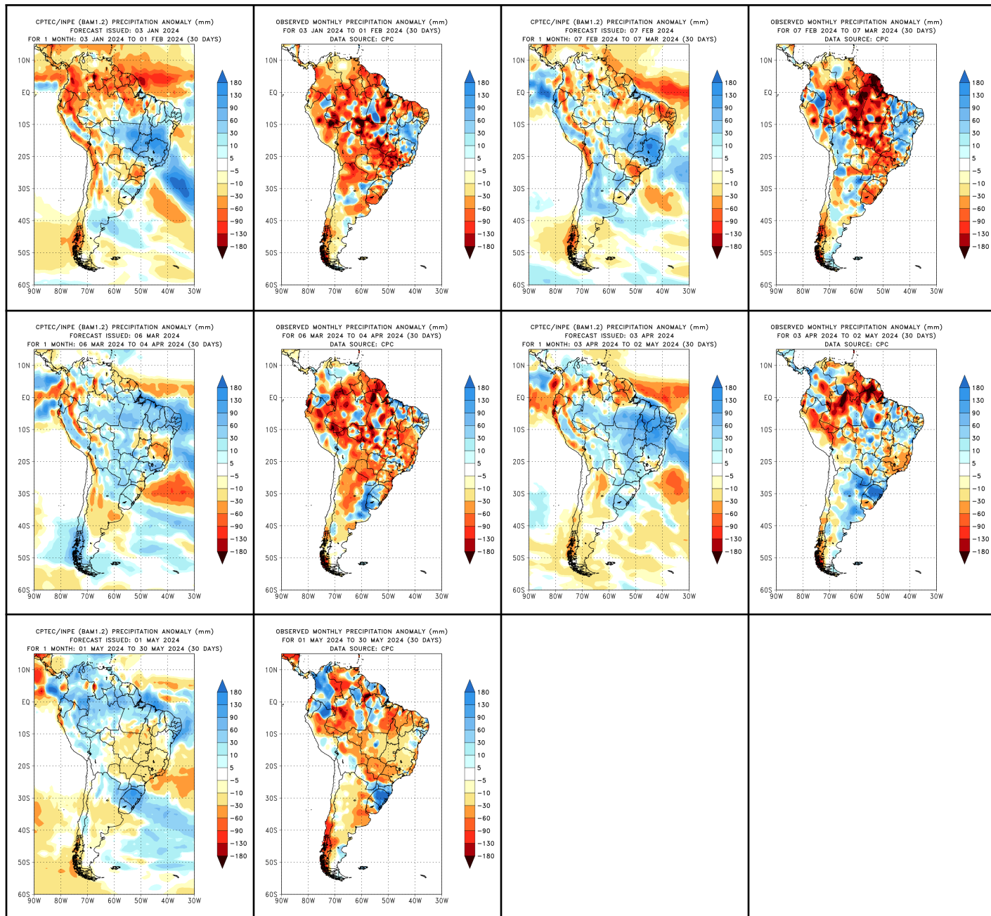
Figura 2.1: Previsão mensal da anomalia de precipitação (BAM-1.2) e suas respectivas observações. Prognósticos inicializados na primeira quarta-feira de cada mês no período de maio de 2023 a maio de 2024.
