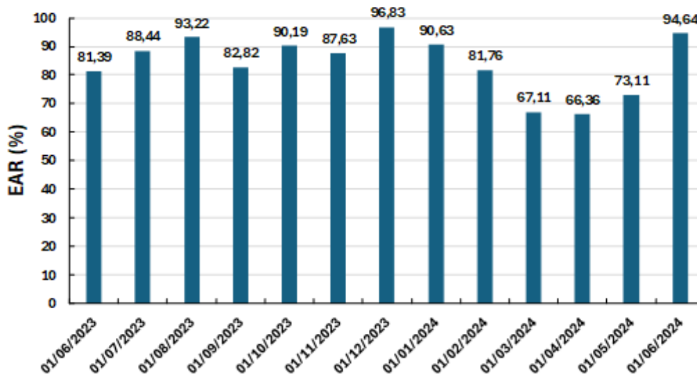
Figura 4.2.2: Evolução do armazenamento dos reservatórios de regularização do subsistema sul entre 01/06/2023 e 01/06/2024.
