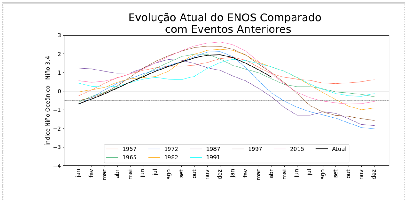
Figura 1.3.2: El Niños fortes e muito fortes ocorridos entre os anos de 1957 e 2024. Fonte: NOAA.
