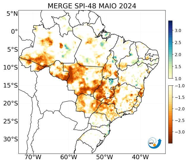
Figura 1.2.1: SPI obtido a partir do MERGE para o período de: a) 1 mês; b) 3 meses; c) 6 meses; d) 9 meses; e) 12 meses; f) 24 meses; g) 48 meses; e h) 60 meses.
