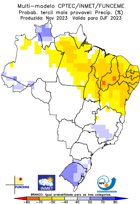
Figura 3.1: Previsão probabilística de precipitação e precipitação observada categorizada para os trimestres SON/23 (a e b) e DJF 23/24 (c e d).
