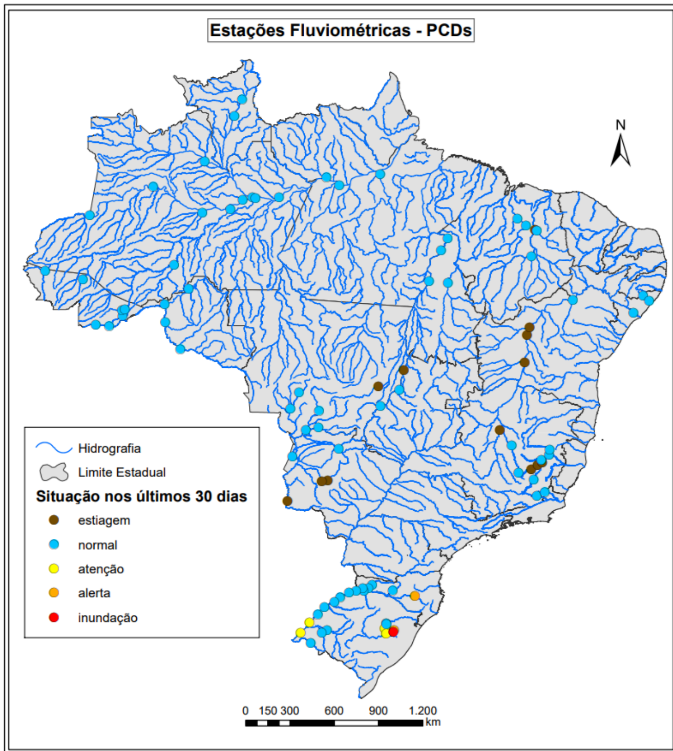
Figura 4.3.1: Situação dos principais rios brasileiros quanto à ocorrência de seca ou cheia observadas nos últimos 30 dias em 91 estações fluviométricas selecionadas.
