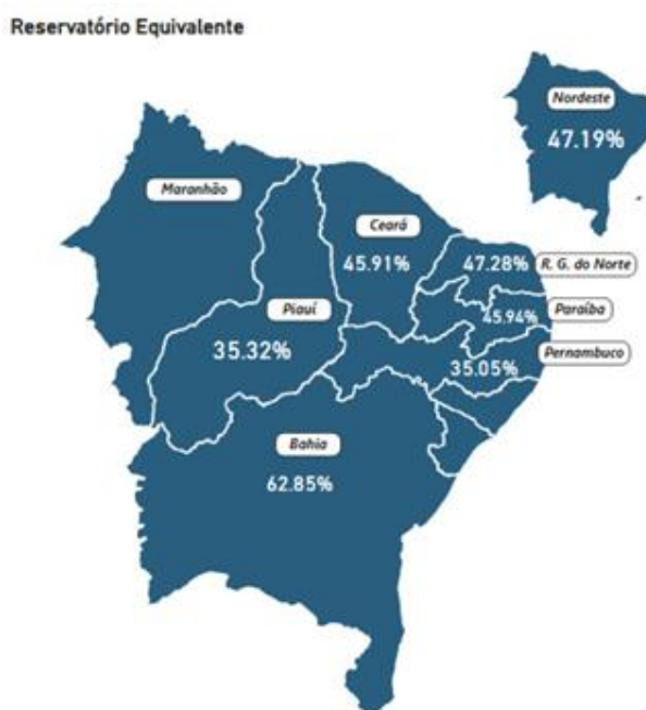
Figura 7: Reservatório Equivalente do Nordeste. Fonte: SAR/ANA.
