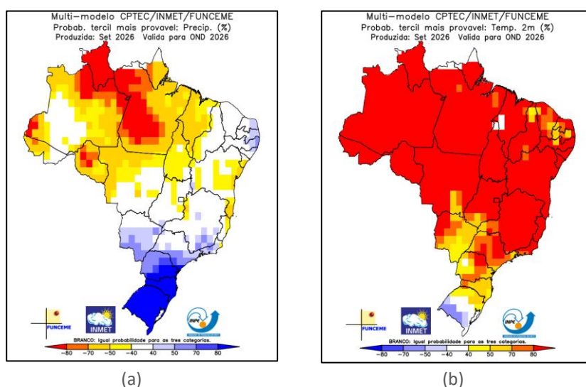
Figura 9: Previsão climática sazonal por tercil (categorias abaixo da faixa normal, dentro da faixa normal e acima da faixa normal), gerada pelo método objetivo (CPTEC/INPE, INMET e FUNCEME). As áreas em branco indicam igual probabilidade para as três categorias. (a) precipitação; (b) temperatura.
