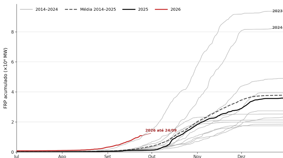
Figura 8: Potência radiativa do fogo (FRP) acumulada dos eventos de fogo no Amapá entre 2014 e 2026. A linha
