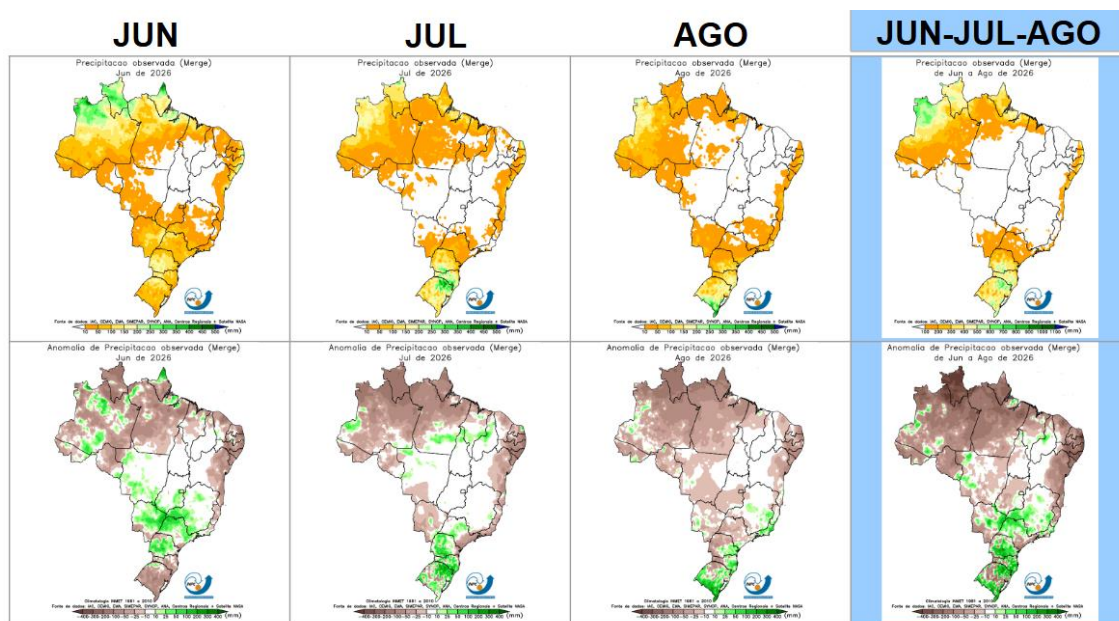
Figura 3: Precipitação e anomalia de precipitação para os meses de junho, julho e agosto de 2026 individualmente e para o trimestre (JJA/2026). Fonte: MERGE/CPTEC-INPE.
