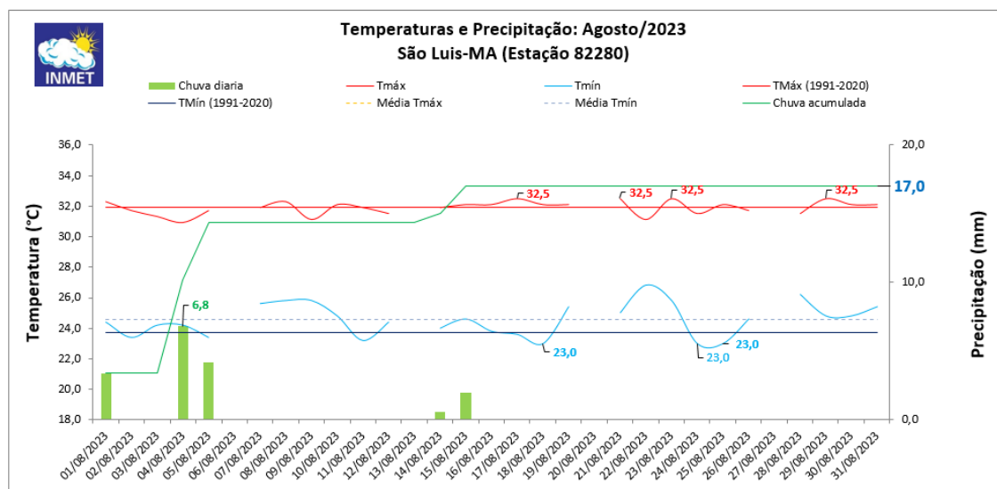
Figura 1: Temperaturas e precipitação (chuva) diárias em agosto de 2023 para São Luís (MA). Referência: Normal Climatológica Inmet (1991 a 2020).
