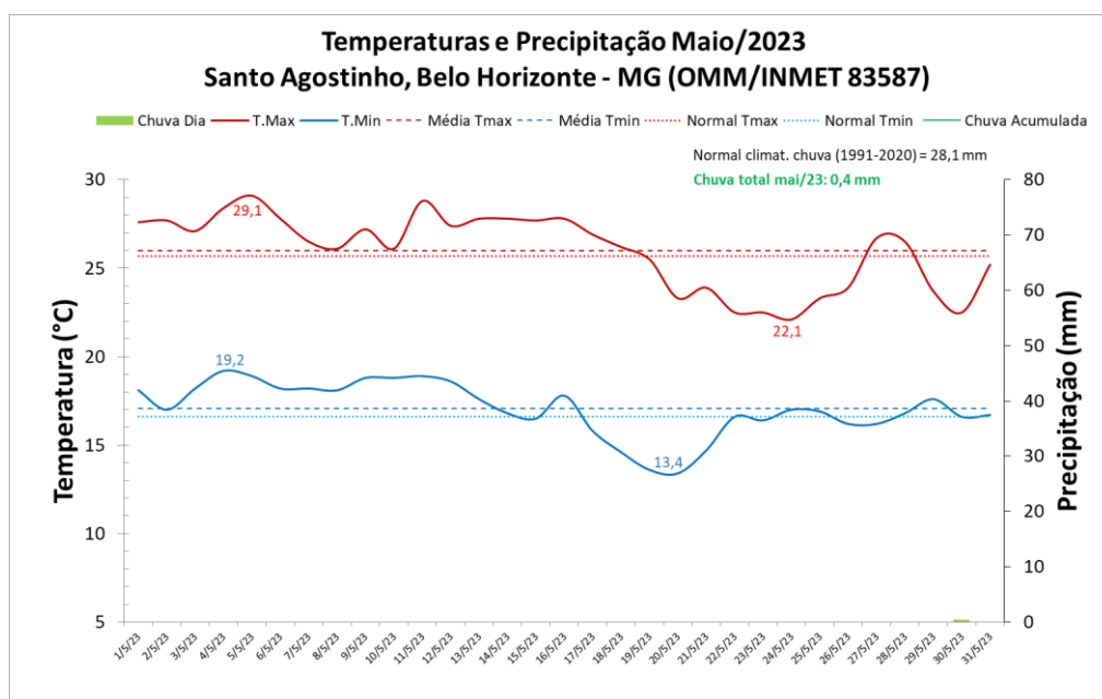
Figura 1: Gráfico contendo as temperaturas máximas, mínimas e precipitação (chuva), da estação convencional, com suas respectivas Normais Climatológicas (1991-2020).
