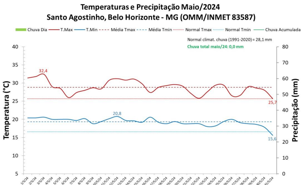
Figura 1: Gráfico com as temperaturas máximas, mínimas e precipitação (chuva) da estação convencional com suas respectivas normais climatológicas (1991-2020).
