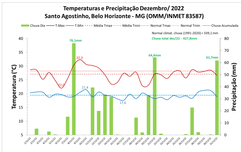
Figura 1 – Gráfico com as temperaturas máximas, mínimas e precipitação, da estação convencional, com suas respectivas Normais Climatológicas (1991-2020).
