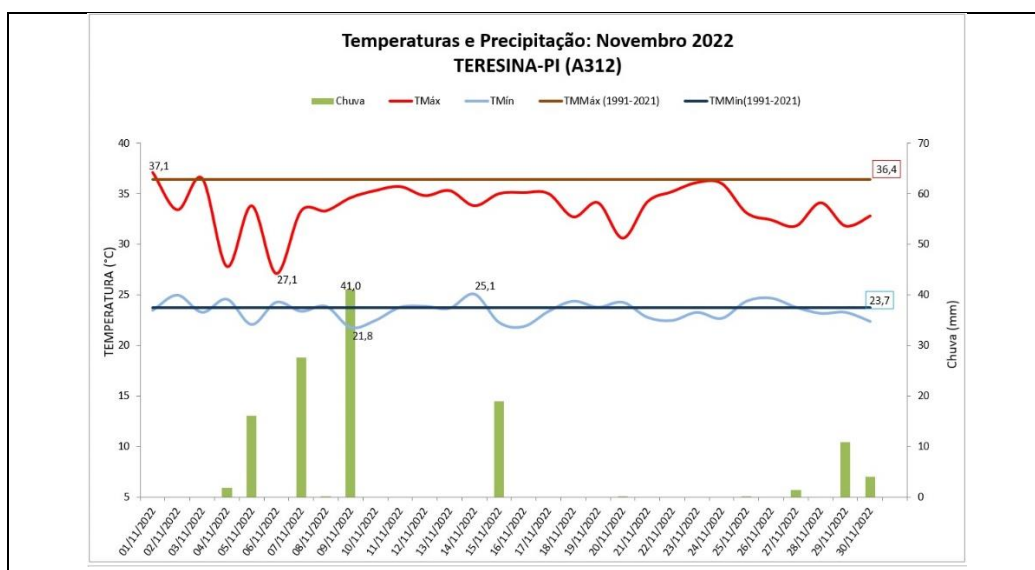
Figura 1 – Gráfico contendo as temperaturas máximas, mínimas e precipitação da estação automática, com suas respectivas climatologias da estação convencional (1991-2020).
