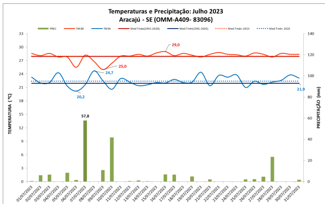
Figura 1: Temperaturas e precipitação (chuva) do mês de julho de 2023, em Aracajú (SE), Média Climatológica (1991-2020).
