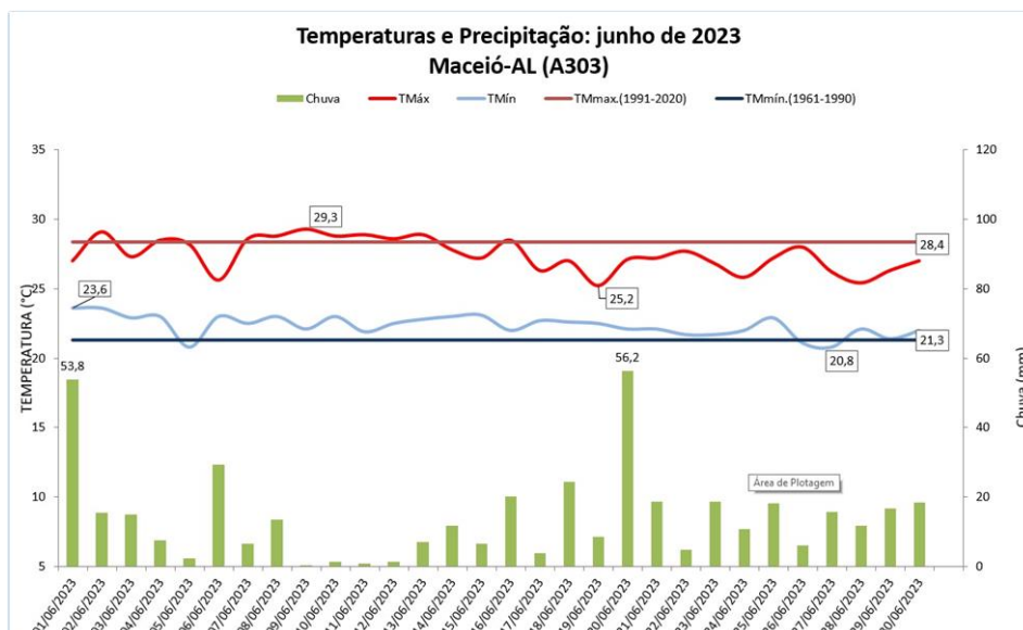
Figura 1– Gráfico com as temperaturas máximas, mínimas e chuva da estação automática do Inmet, com suas respectivas séries climatológicas da estação convencional (1991-2020 e 1961-1990).
