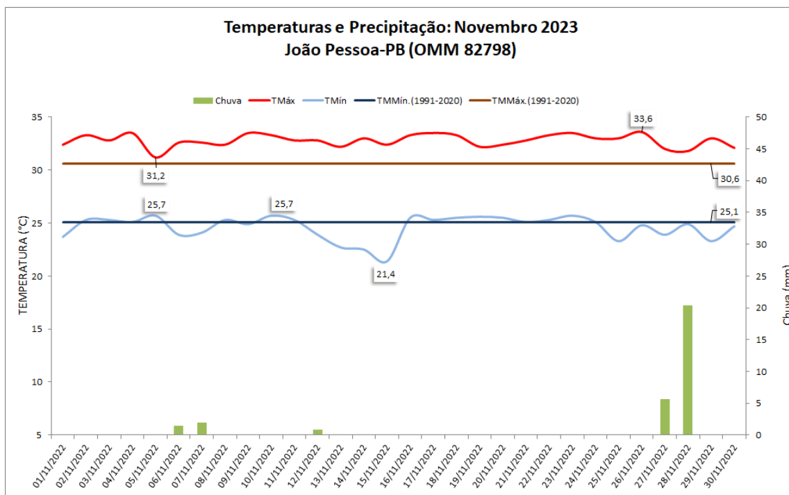
Figura 1: Gráfico com valores de temperatura máxima e mínima e precipitação (chuva) na estação convencional, com suas respectivas Normais Climatológicas (1991-2020).
