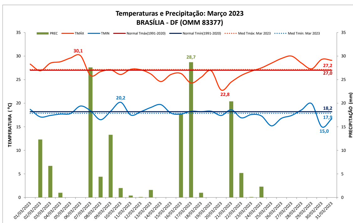
Figura 1: Temperaturas e precipitação (chuva) de março de 2023 em Brasília (DF). Normal Climatológica 1991/2020.
