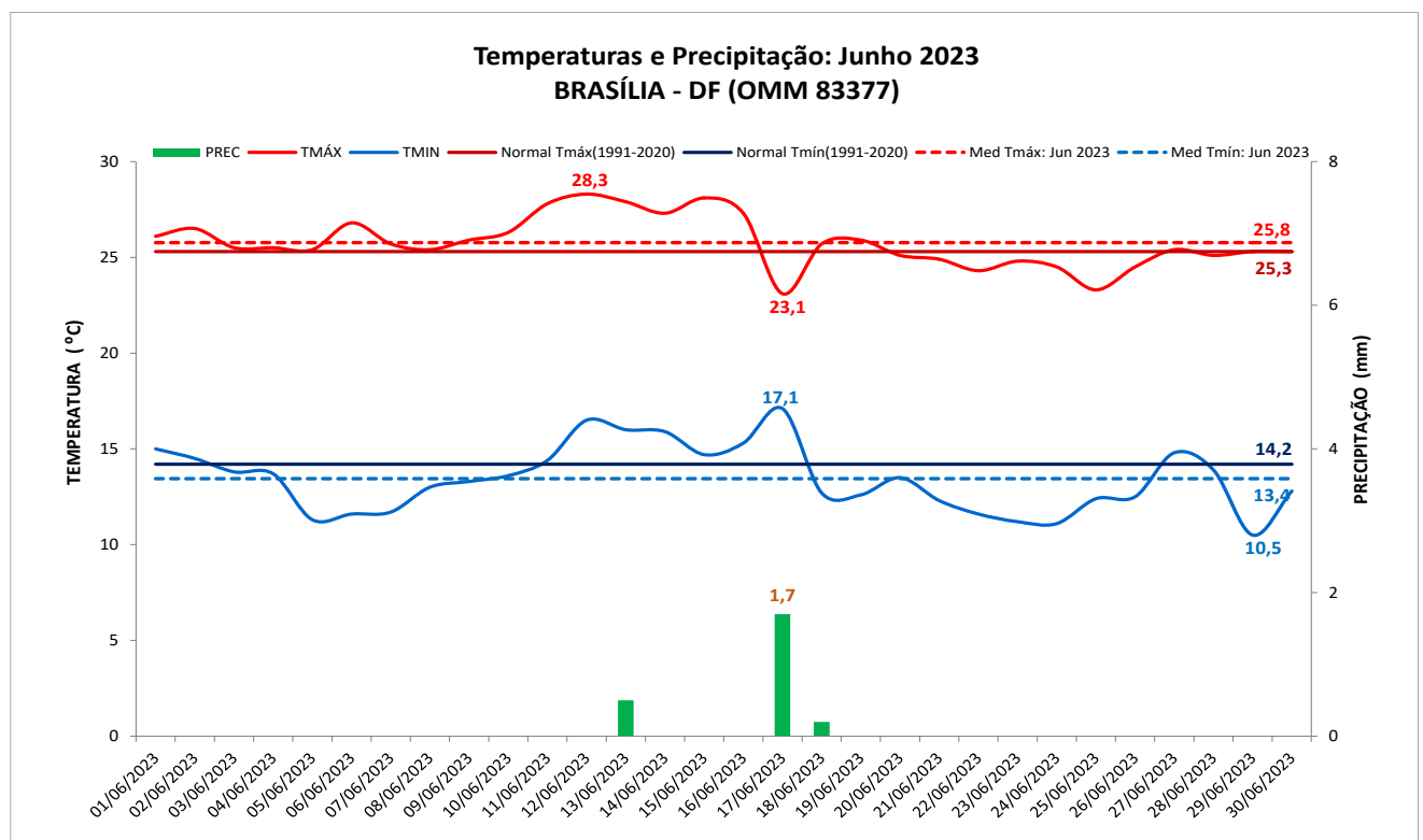
Figura 1: Temperatura e precipitação (chuva) do mês de junho de 2023 em Brasília (DF).
