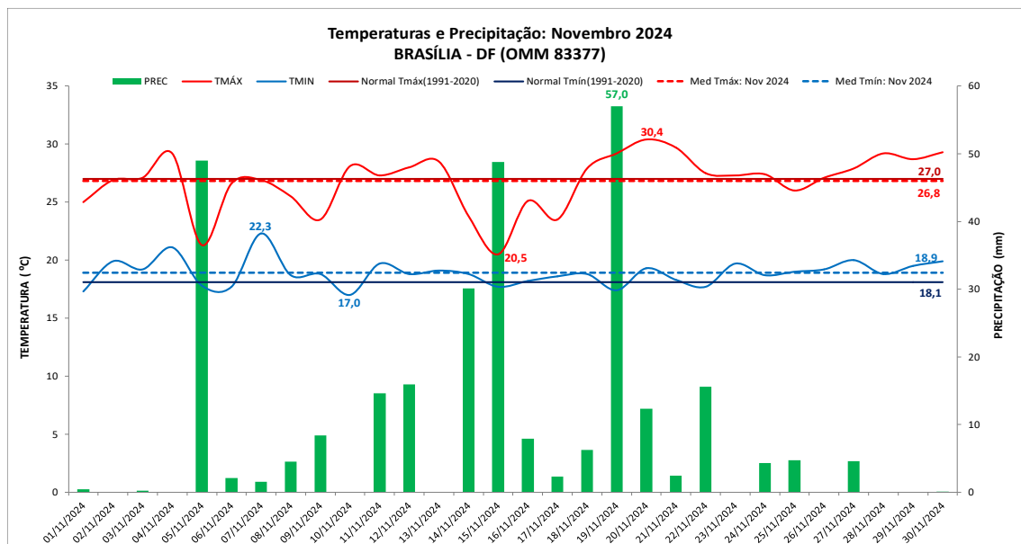
Figura 1: Temperaturas e precipitação do mês de novembro de 2024 em Brasília – DF versus a Normal Climatológica (1991 a 2020)
